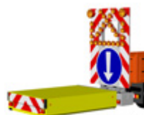
Pojízdné tlumiče nárazu TMA
